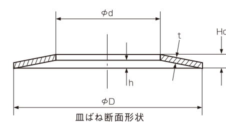
BDS (注) 表中内径の ( ), (( )) はそれぞれ呼びの ' ' に対する内径を示す。 単位 mm
